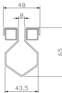
coupe a fente pour piscines
