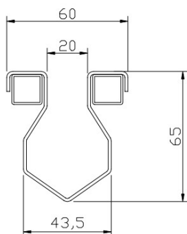
przekrój standardowy
